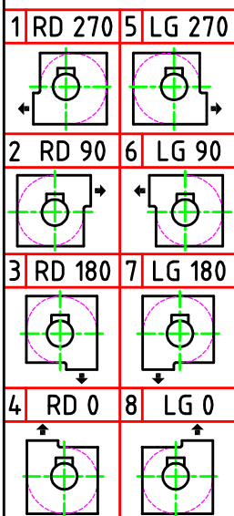
ORIENTATIONS COTE MOTEUR
