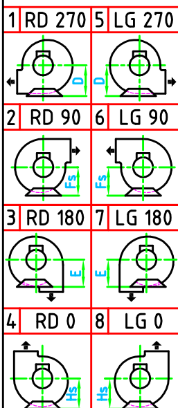
ORIENTATIONS COTE MOTEUR
