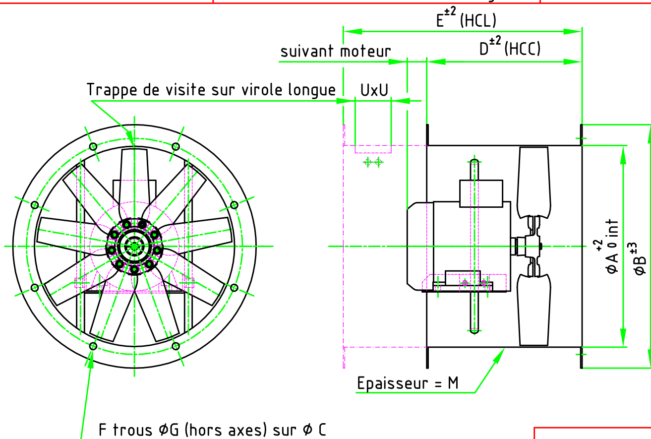
DEFINITION SUIVANT PLAN TABLEAU N° 21236
